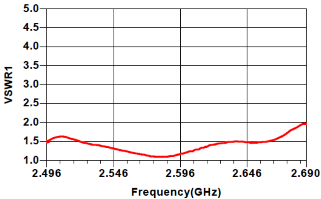
S11 VSWR
